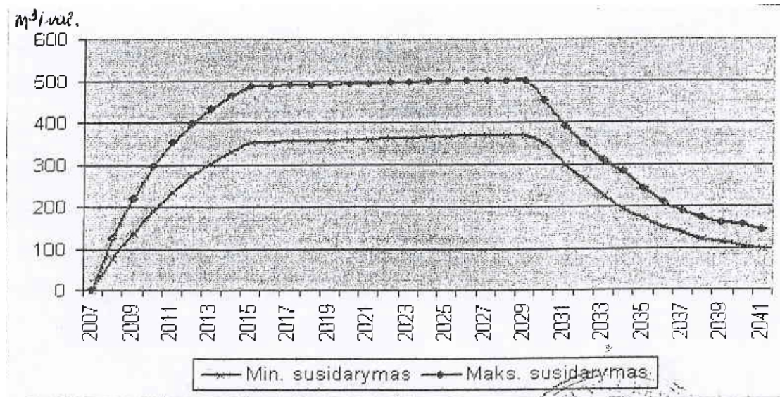
1 pav. Prognozuojamas sąvartyno dujų susidarymas
